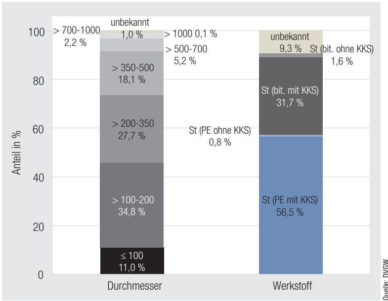
Abb. 5: Aufteilung der Leitungen der Verteilnetzbetreiber >16 bar in Prozent
