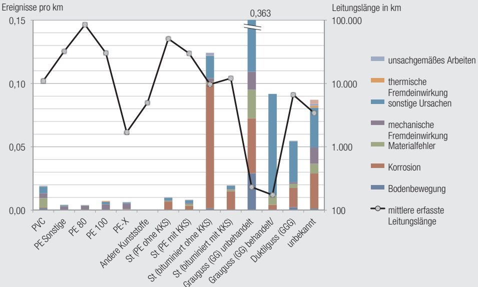
Abb. 14: Ereignisse pro km für Leitungen der Verteilnetzbetreiber < 16 bar nach Werkstoff und Ursache
