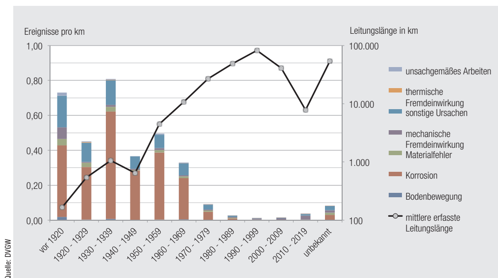
Abb. 12: Ereignisse pro km Leitungen der Verteilnetzbetreiber \leq 16 bar nach Altersgruppe und Ursache
