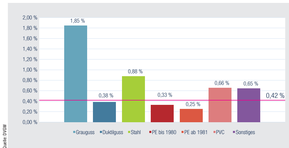
Abb. 5: Rehabilitationsrate von Anschlussleitungen nach Werkstoffen
